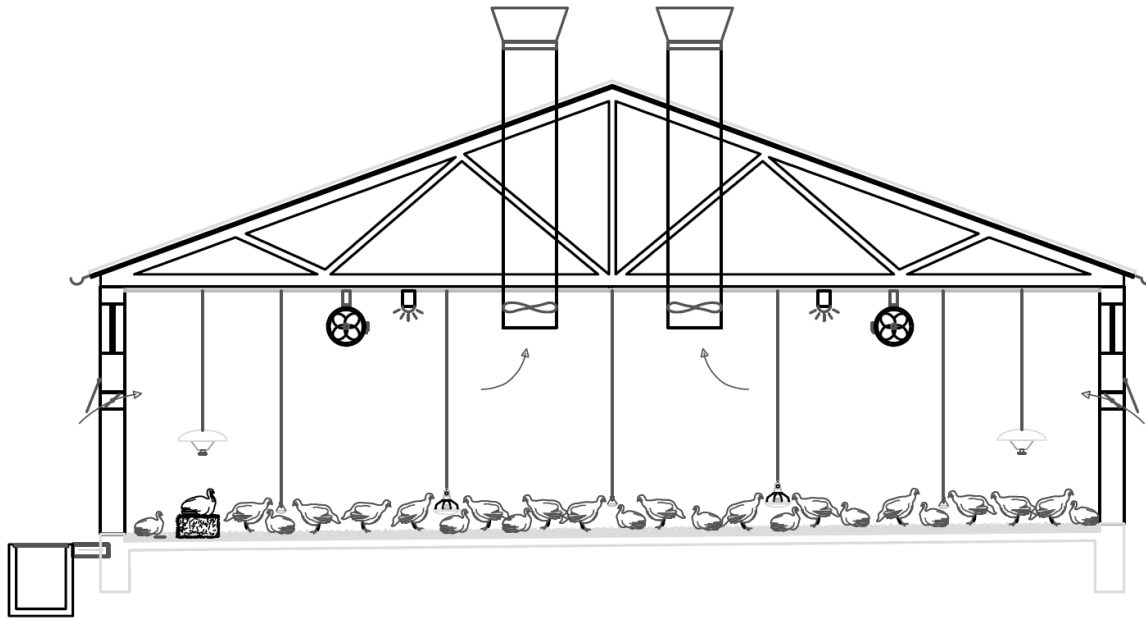
Abb. 1: Skizze des Haltungsverfahrens
