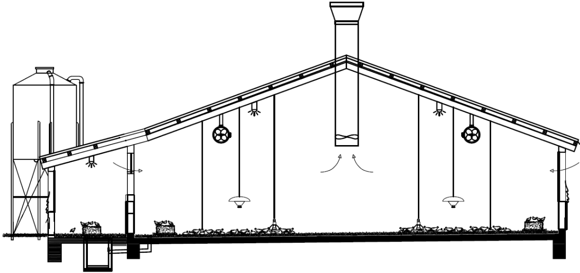
Abb. 1: Skizze des Haltungsverfahrens
